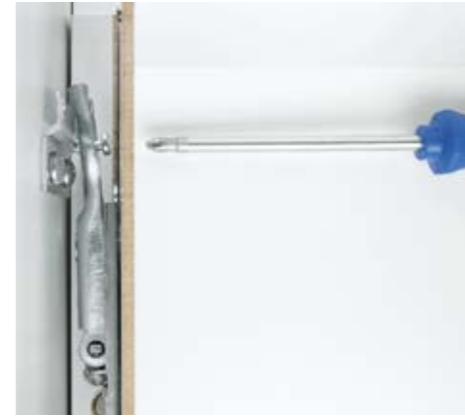
Verdeckte Schrankaufhängung mit Sicherungsschraube Concealed cabinet mounting with lock screw Enganche de mueble oculto con tornillo de seguridad
